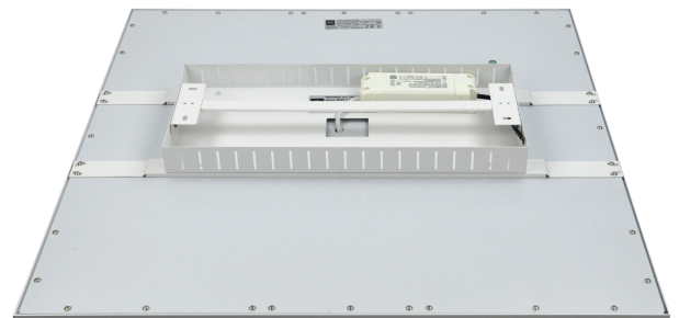
Montagerahmen für Anbau-Montage
